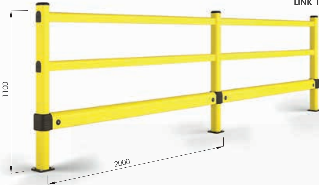
LINK 120/1
