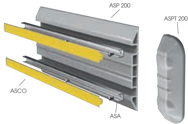
ASP 200
