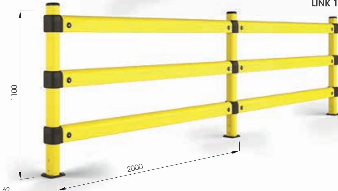
LINK 120/3
